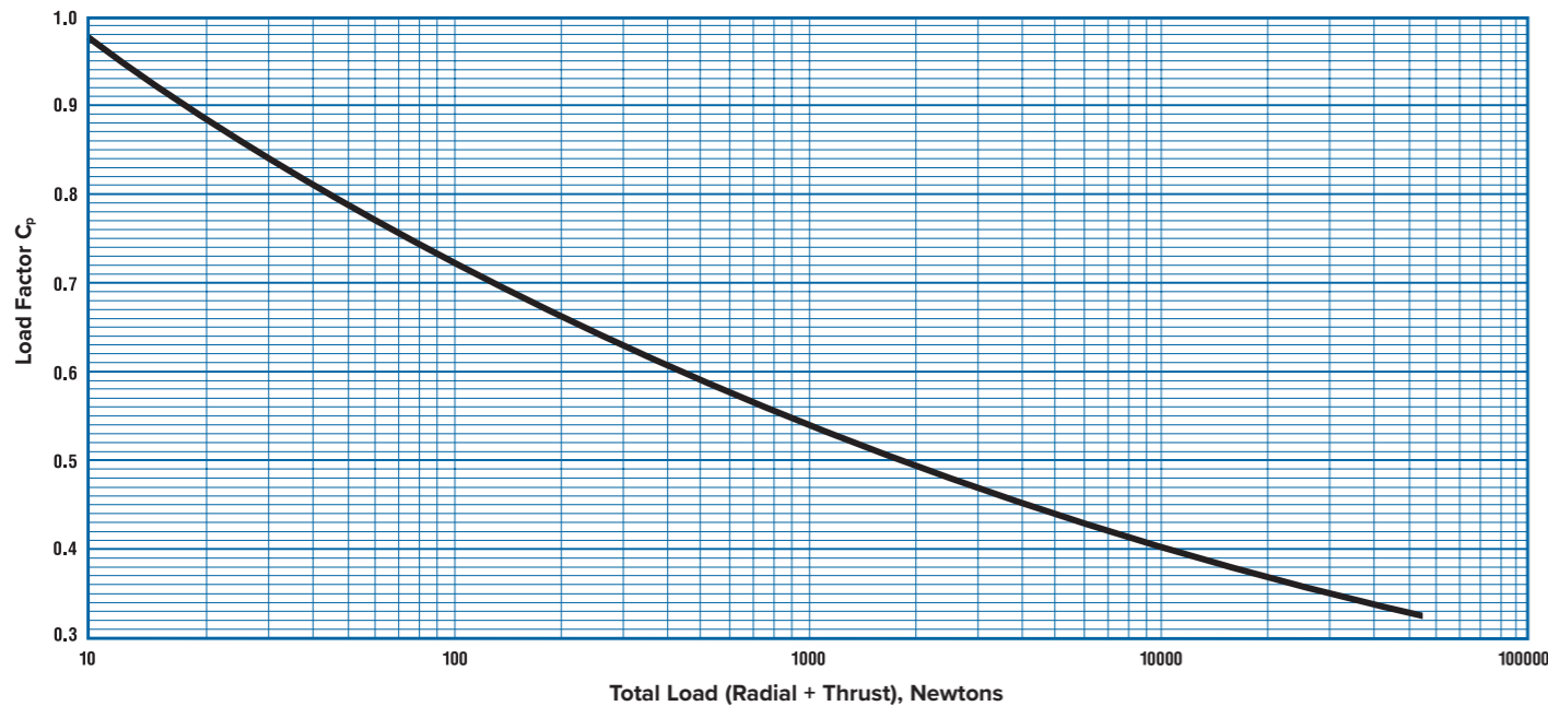
Fig. 19. Load factor Cp.
