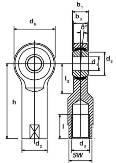
SI..E Internal Thread
